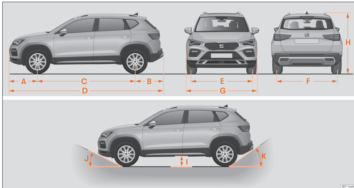
Fig. 236 Dimensiuni.
