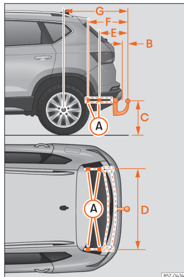
Fig. 185 Limite și puncte de fixare pentru montarea ulterioară a unui dispozitiv de remorcă.
