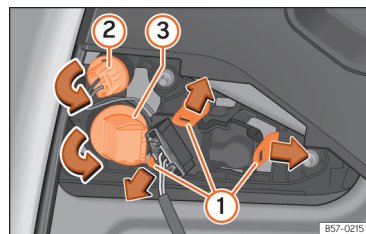
Fig. 206 scoaterea soclului becului.
