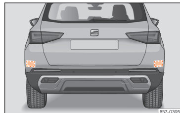
Fig. 108 Autovehiculul văzut din spate: suprafețele cu senzori radar.
