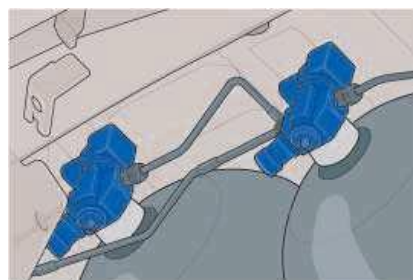
Supapele electromagnetice de închidere de pe rezervoarele de gaz
