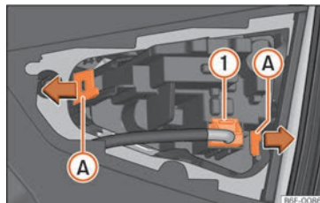
Fig. 174 scoaterea soclului becului.
