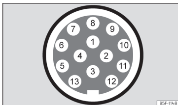
Fig. 149 Diagramă: alocarea pinilor prizei electrice a remorcii.
