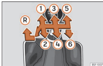
Fig. 84 Schema de schimbare a treptelor de viteză la cutia de viteze manuală cu 5 sau 6 trepte.
