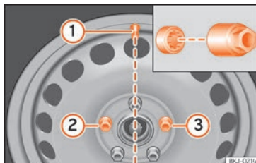
Fig. 197 Înlocuirea unei roți: ventilul anvelopei ① și poziția corectă a șurubului de blocare antifurt al roții ② sau ③.
