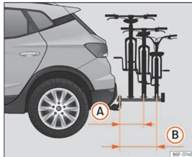
Fig. 151 Reprezentare schematică a ieșirii maxime în consolă a unui suport de biciclete pentru două sau trei biciclete.
