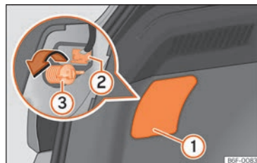
Fig. 171 Portbagaj: accesul la șurubul care fixează ansamblul lămpii spate.
