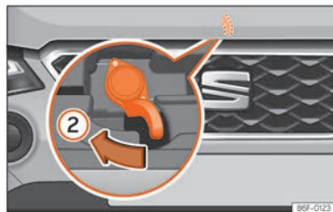
Fig. 179 Manetă sub capotă.
