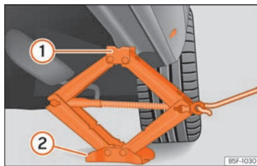
Fig. 199 Traversa: montarea cricului pe autovehicul.
