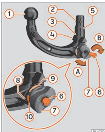
Fig. 154 Prezentare generală: cârlig de remorcă detașabil.
