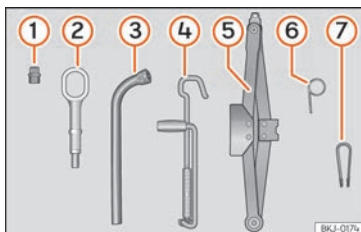
Fig. 157 Sub podeaua portbagajului: trusa de scule.
