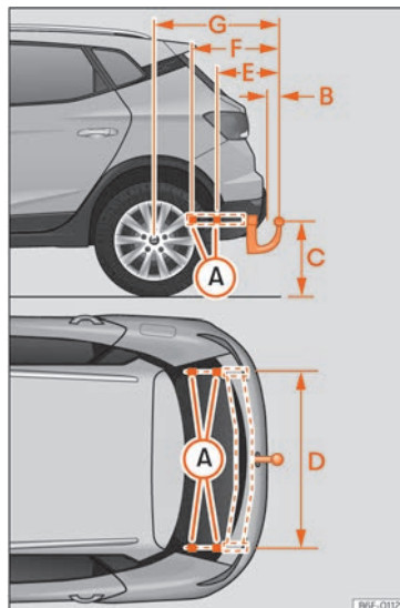
Fig. 152 Limite și puncte de fixare pentru montarea ulterioară a unui dispozitiv de remorcare.
