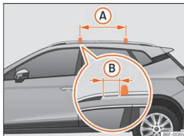
Fig. 148 Punctele de prindere pentru barele transversale pentru suportul pentru portbagajul de acoperiș
