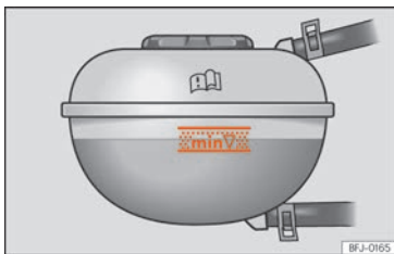
Fig. 180 În compartimentul motor: marcajul de pe vasul de expansiune al lichidului de răcire.
