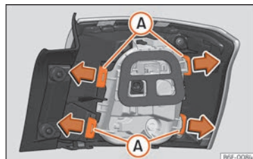
Fig. 172 Clemele de fixare pe partea din spate a lămpii spate.
