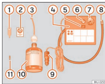
Fig. 201 Afișajul standard: componentele kitului de reparație anvelope în caz de pană.
