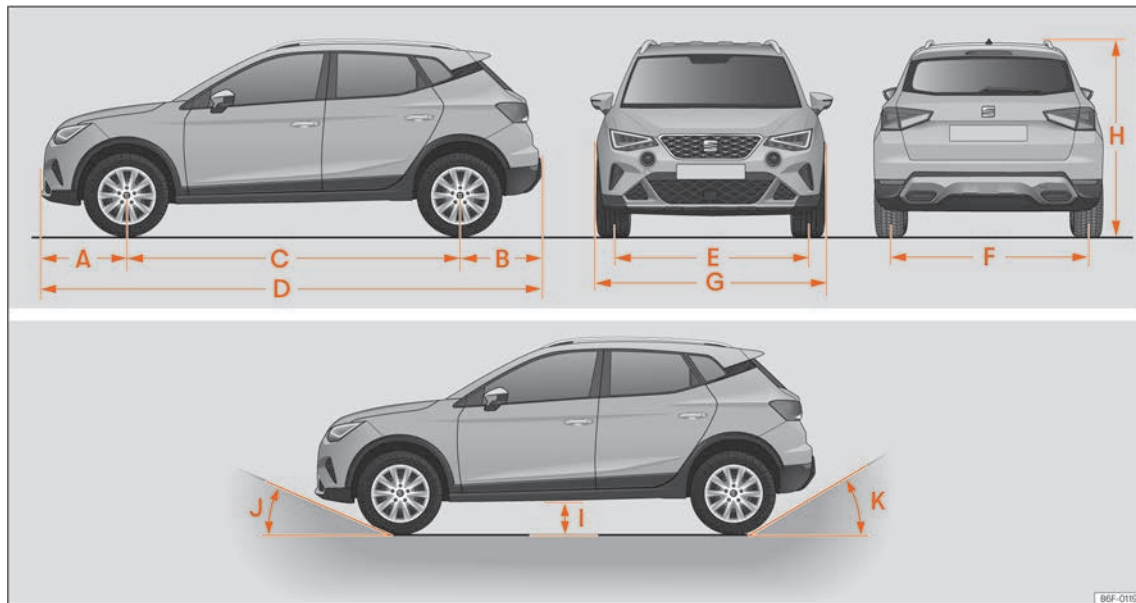
Fig. 206 Dimensiuni și unghiuri.
